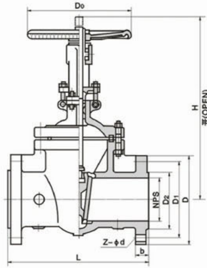
主要外形和连接尺寸 Main External and Connection Dimension
