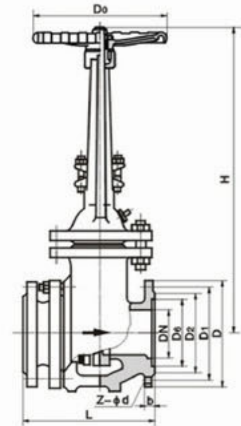
主要外形和连接尺寸(mm)Main External and Connection Dimension
