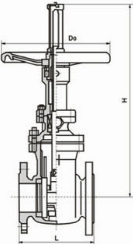
ZBPZ44Y自动补偿平板闸阀
