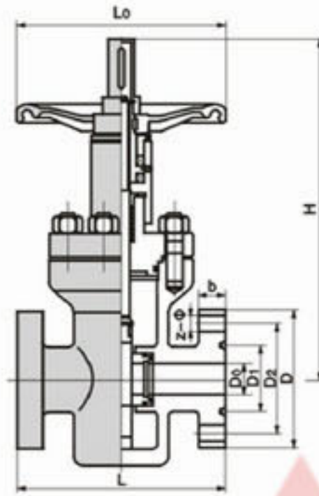
GPZ43Y油田专用高压平板闸阀
