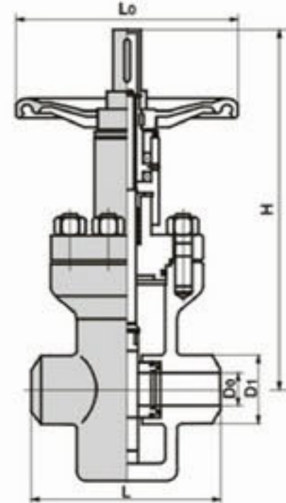
GPZ63Y油田专用高压平板闸阀
